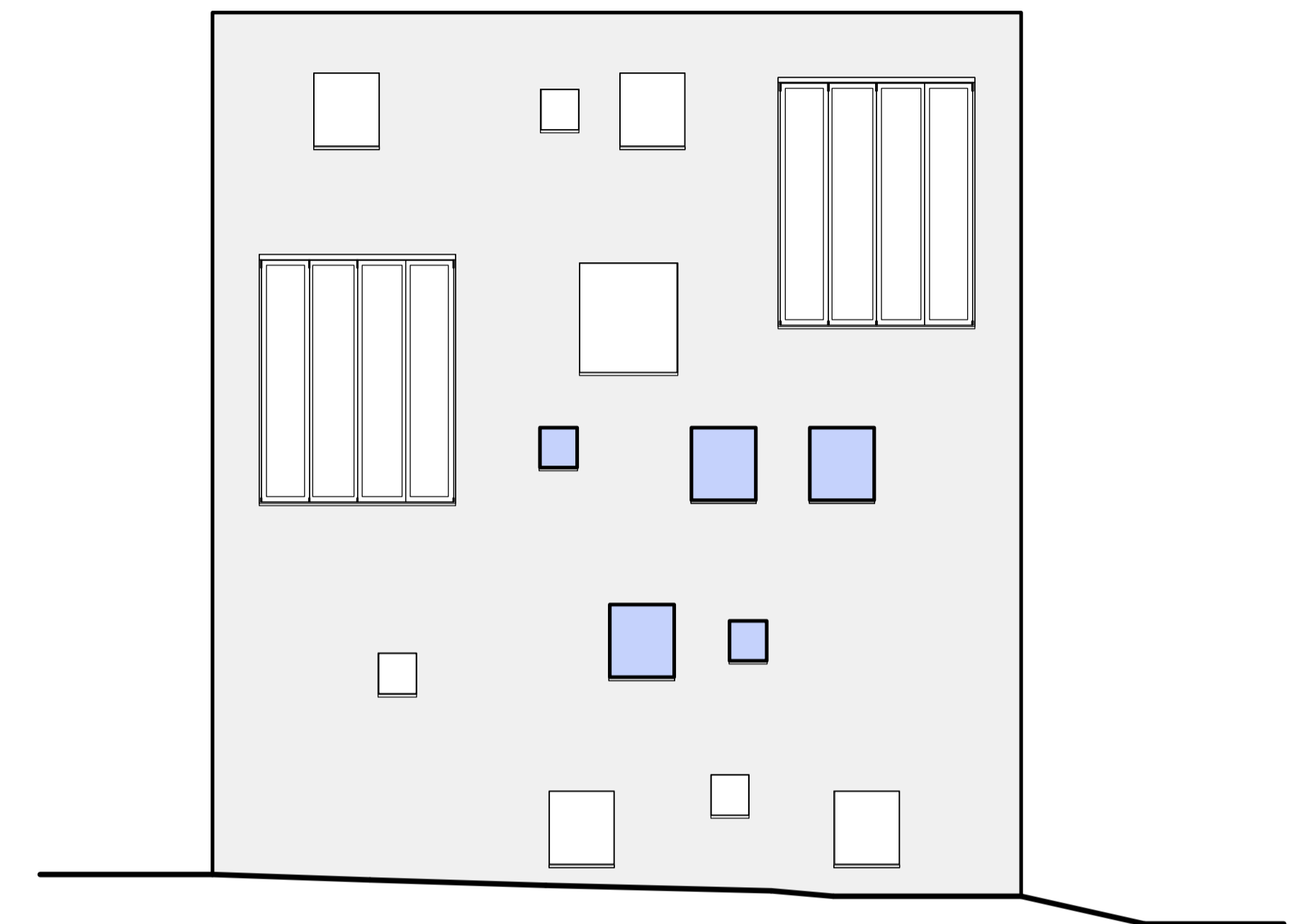
ZIJGEVEL LINKS
