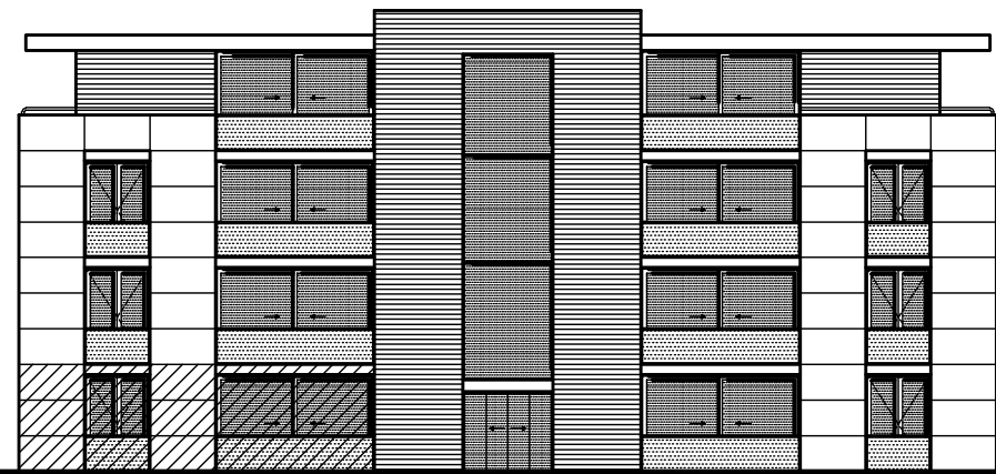
voorgevel gebouw 1
