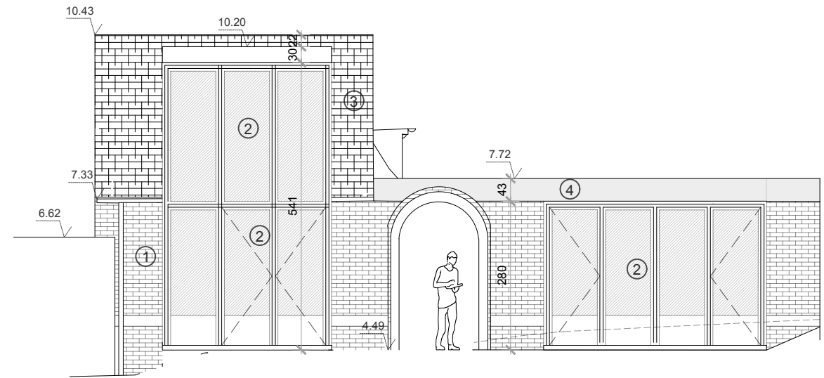
Z-W gevel
