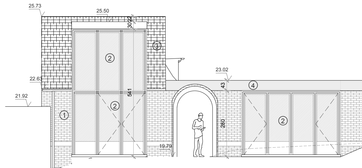
Z-W gevel
