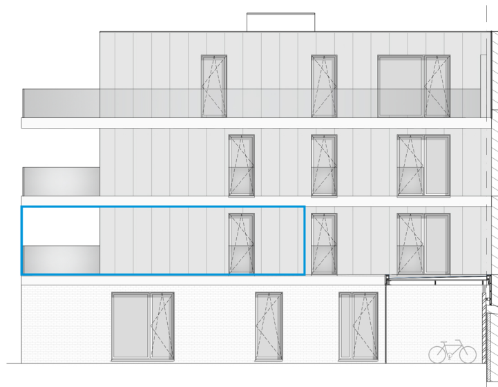
Achtergevel
