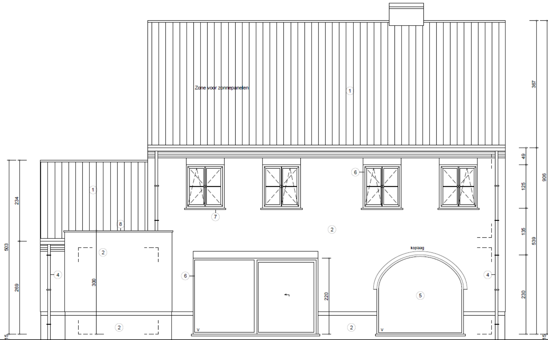
Achtergevel
