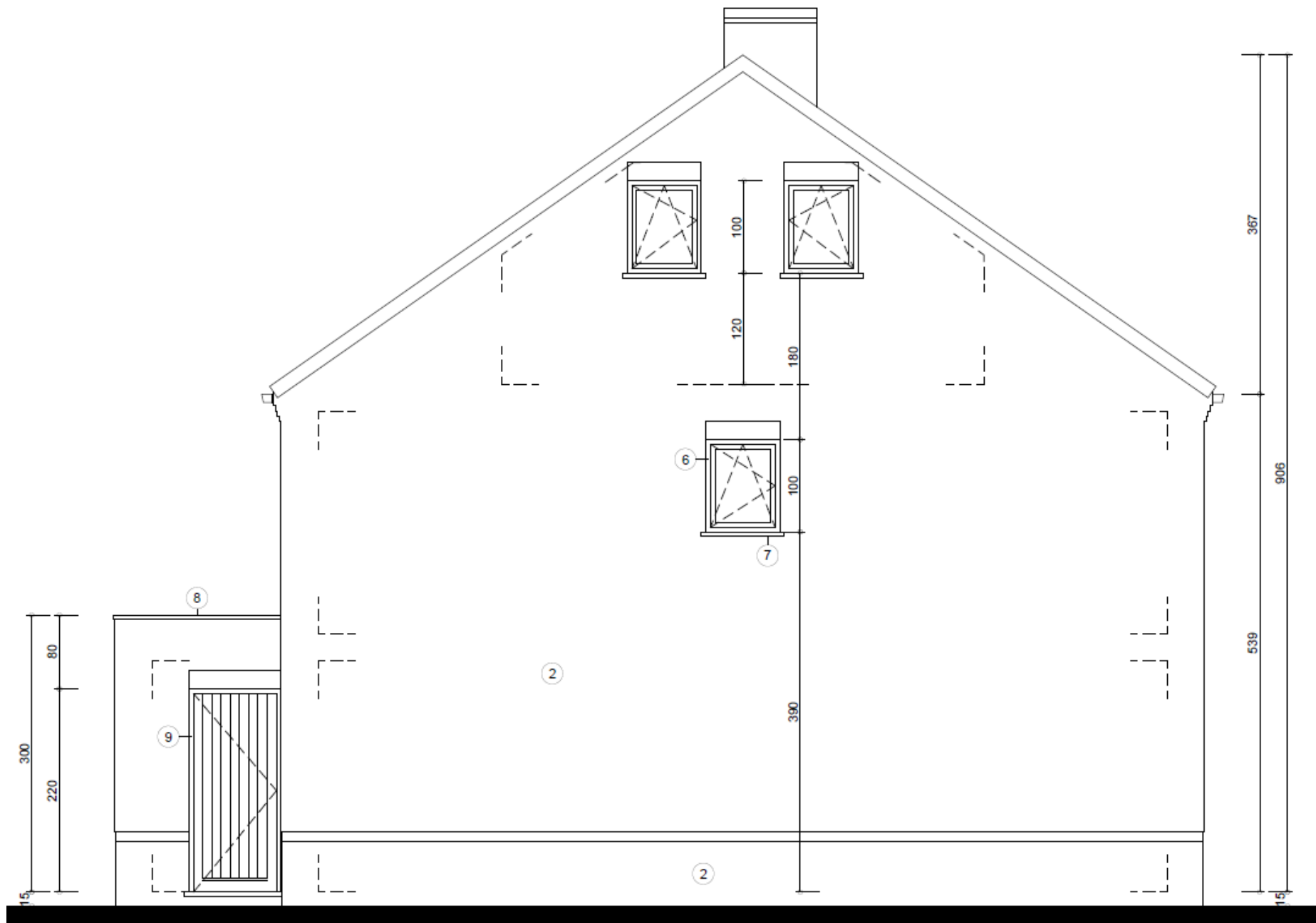
Zijgevel links
