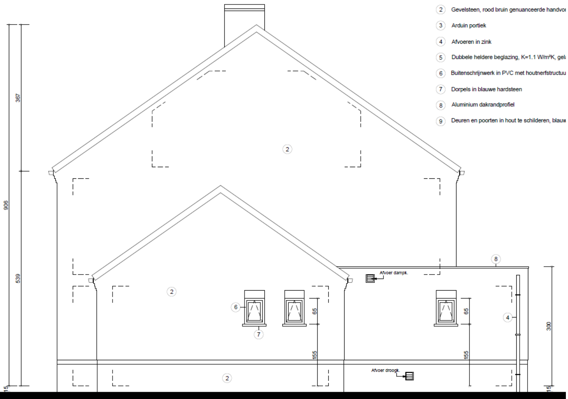
Zijgevel rechts
