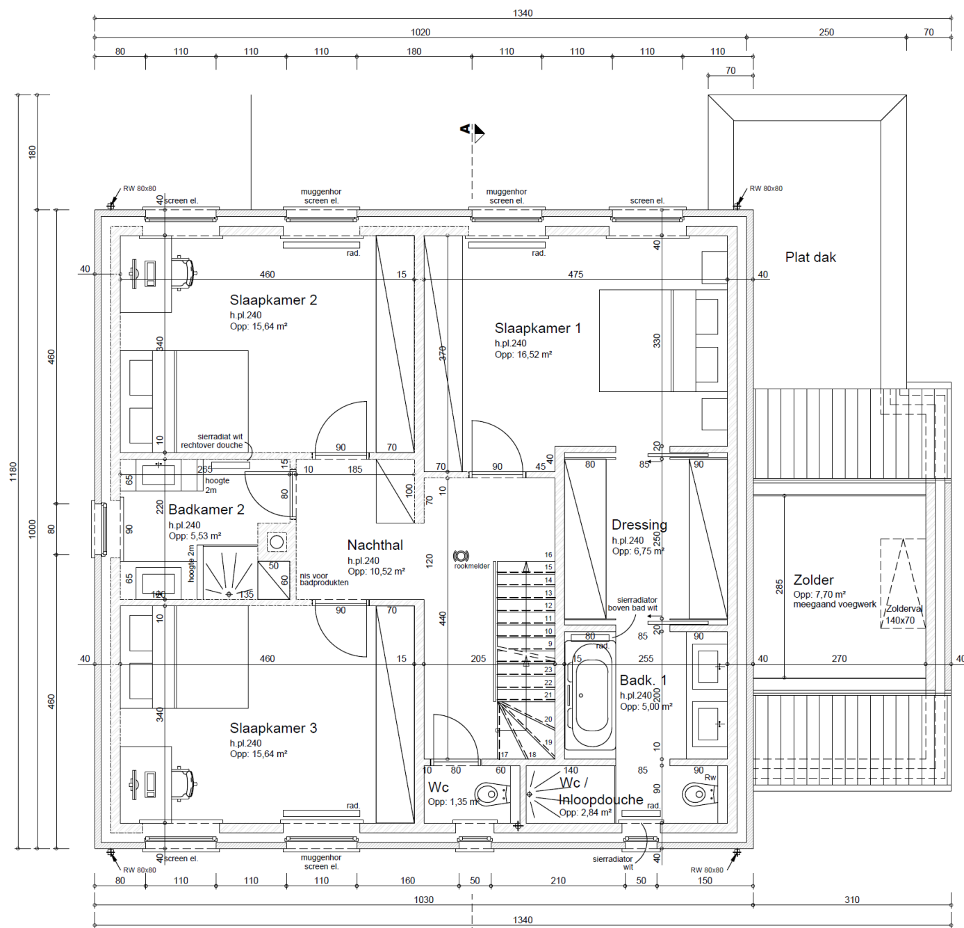
Verdiepingsplan
