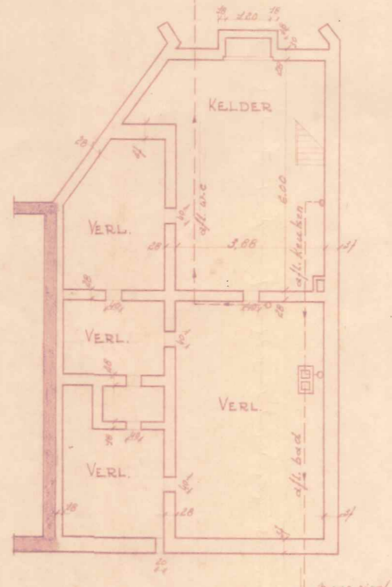
KELDERING
