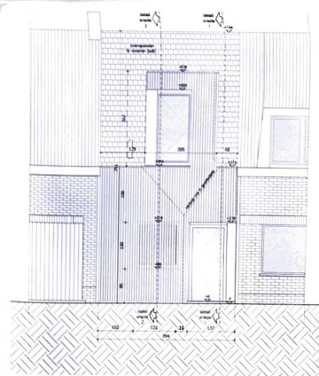
VOORGEVEL
