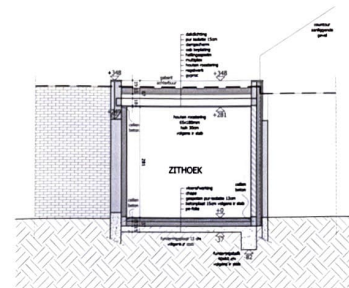
SNEDE DD'
