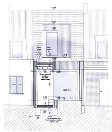
ACHTERGEVEL (SNEDE BB')
