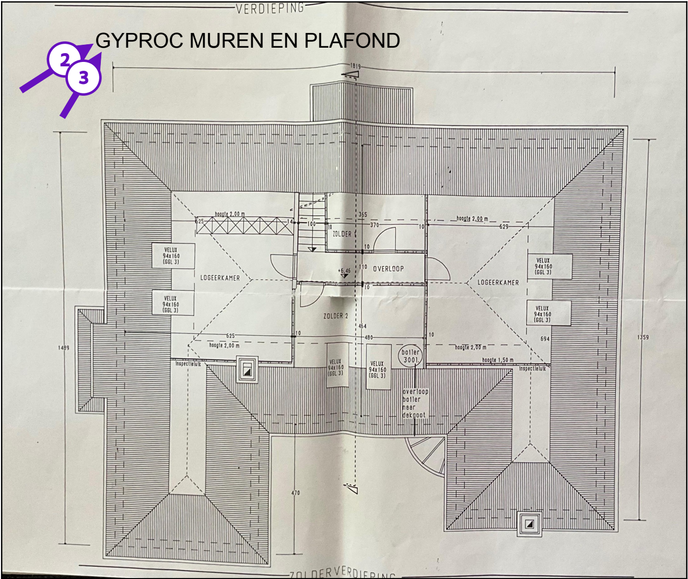
Legende van plan 1.4: zolderverdiep
