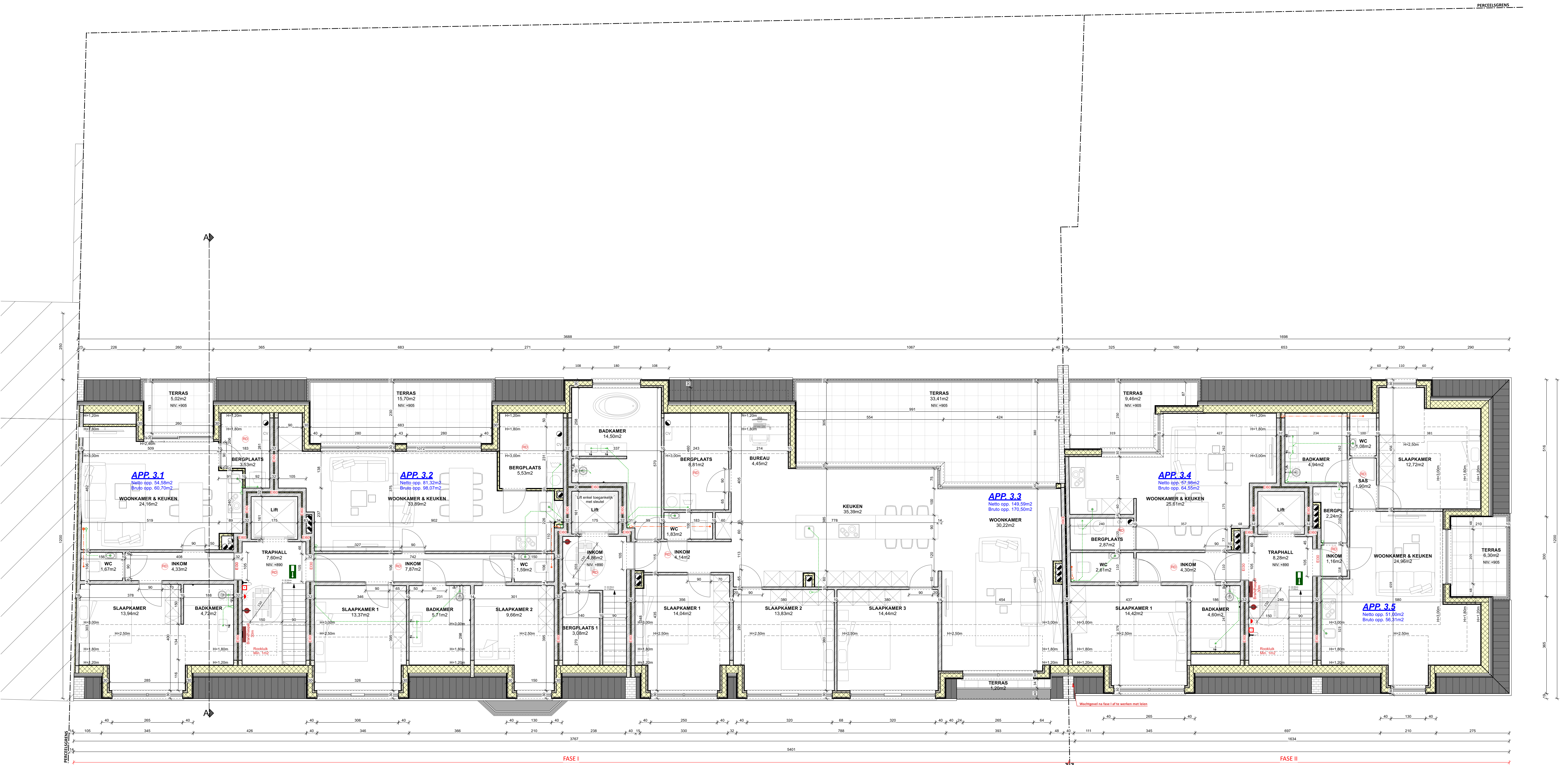
VERDIEPING +3 Schaal 1/50
