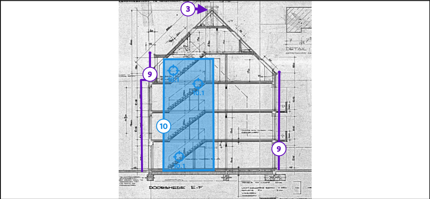
Legende van plan 1.2: doorsnede
