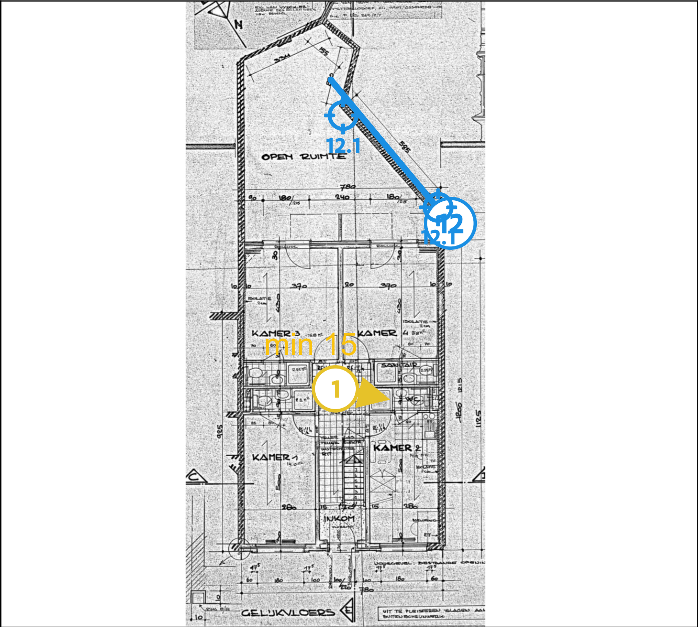
Legende van plan 1.4: niveau 0
