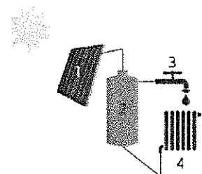
1 Zonnecollector | 2 Opslagvat zonnecollector | 3 Sanitair warm water | 4 Algemeen element voor ruimteverwarming (radiator)
